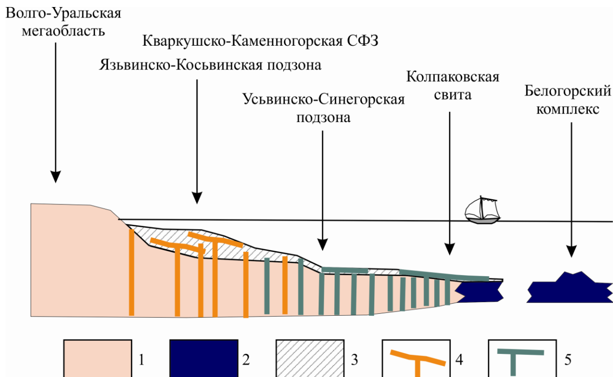
Рис. 4. Схема геологического строения позднепротерозойской рифтогенной пассивной континентальной окраины.
