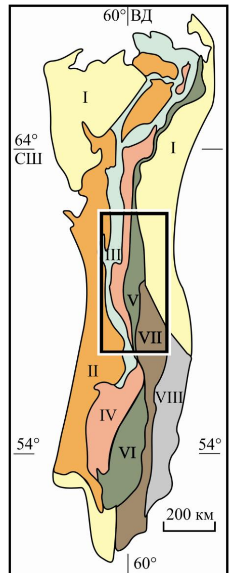
Рис. 1. Схема структурно-формационного районирования Урала.
