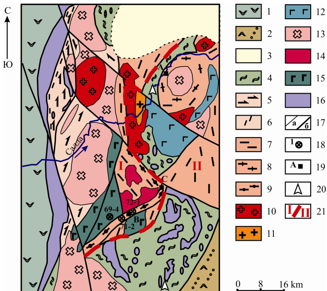
Рис. 8. Геологическая схема Салдинского метаморфического комплекса (составлена по материалам геологических съемок УГСЭ под руководством автора, с упрощениями).
