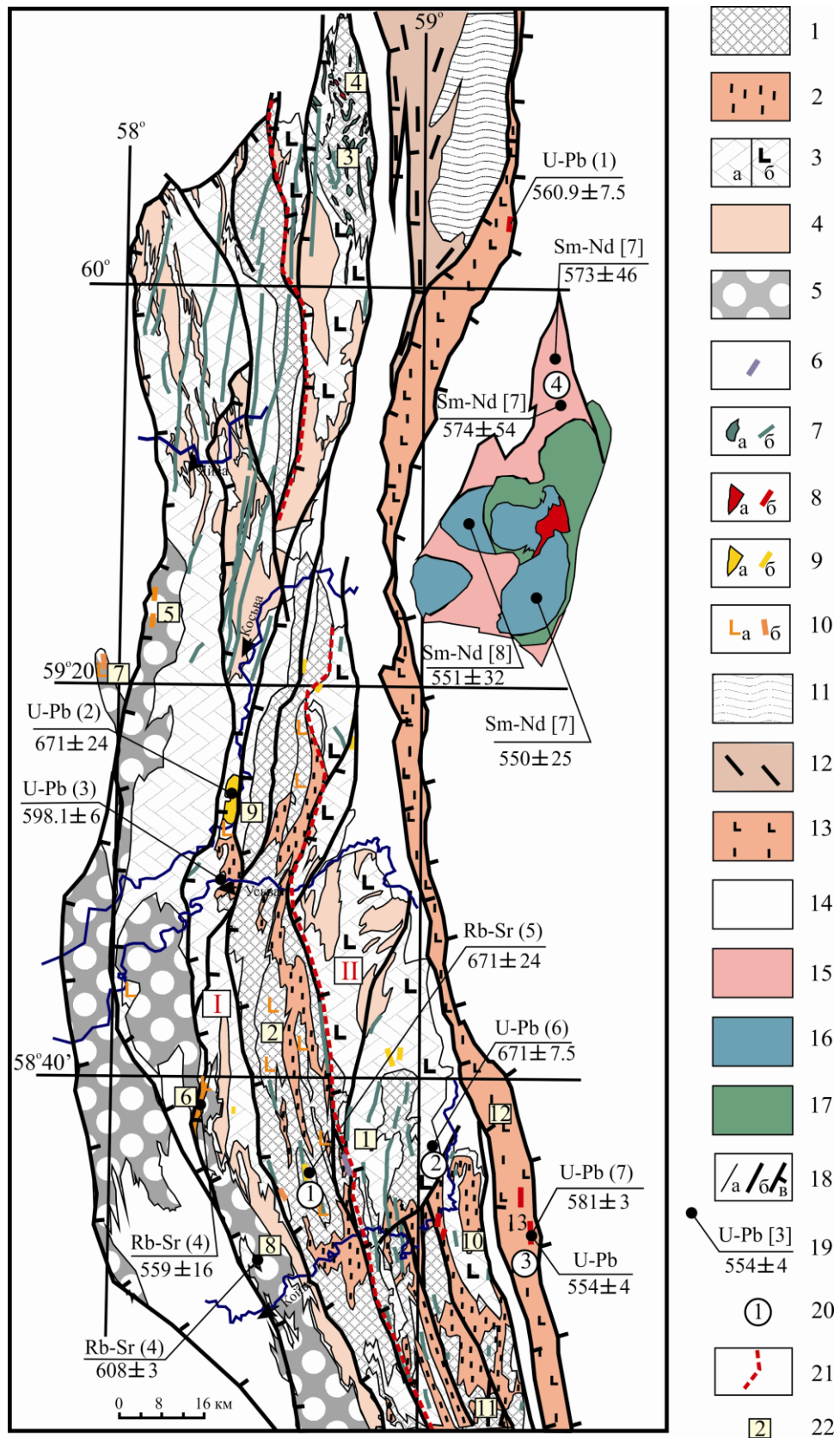
Рис. 2. Схема геологического строения Кваркушко-Каменногорской структуры и её обрамления (составлена с привлечением материалов В.Я. Алексеева, И.В. Короткова, С.Б. Суслова, Л.И. Десятниченко, В.В. Генералова, В.В. Шалагинова).
