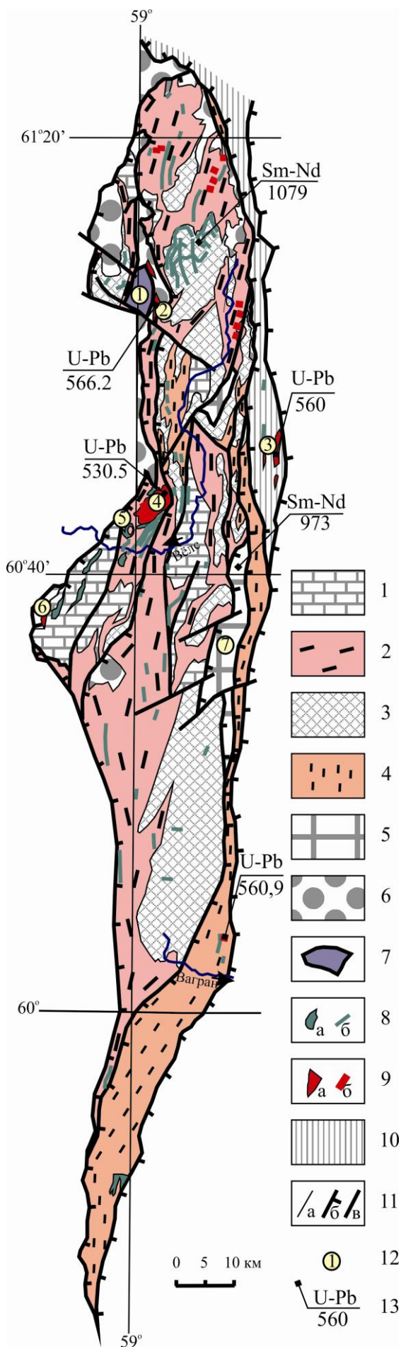
Рис. 5. Схема геологического строения Ишеримской структуры.
