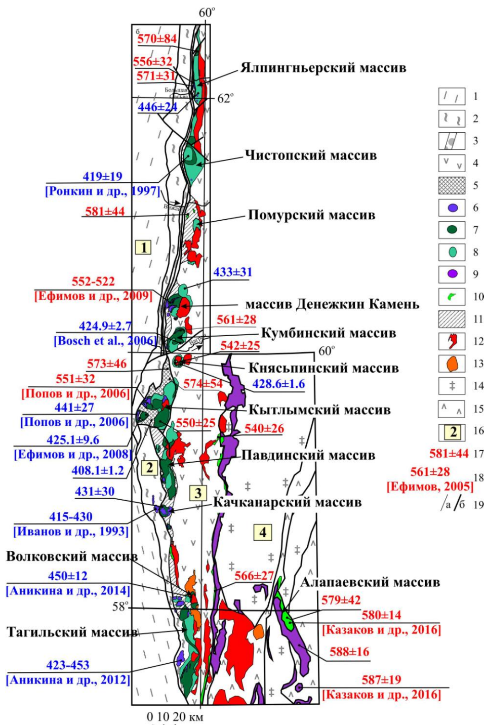
Рис. 7. Схема размещения докембрийских магматических и метаморфических комплексов на восточном склоне Среднего и Северного Урала.
