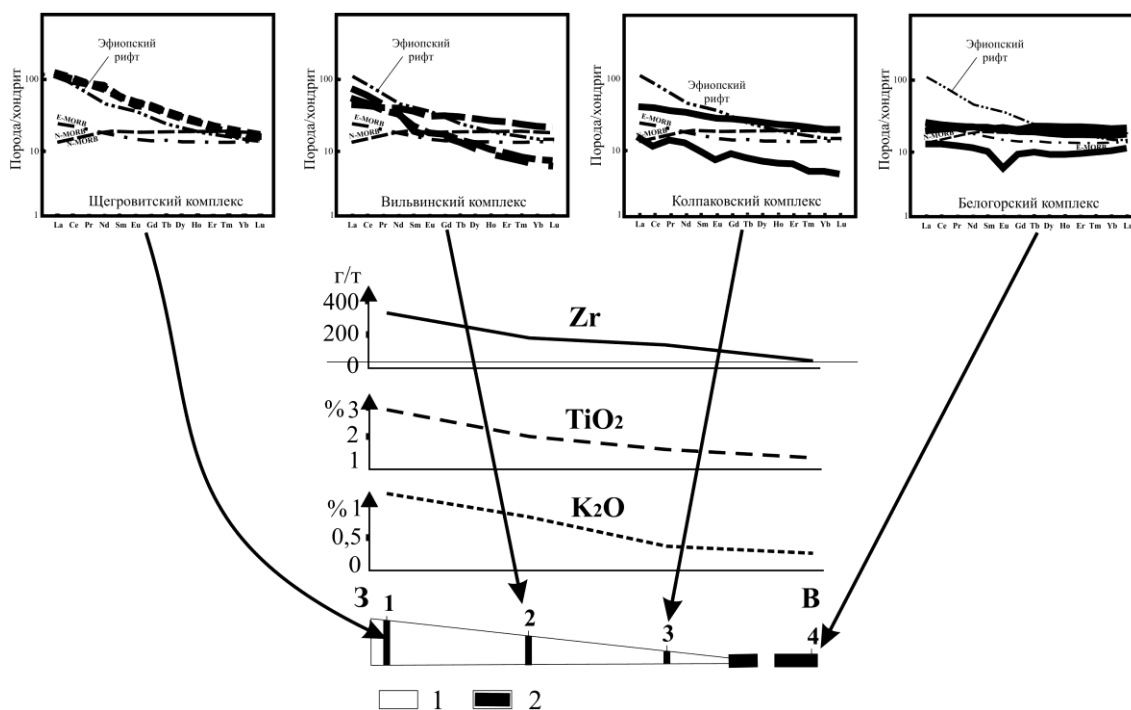
Рис. 3. Геохимическая зональность допалеозойских магматических образований Кваркушского антиклинория и его восточного обрамления. Земная кора континентального (1) и океанического или островодужного (2) типов
