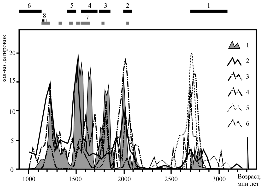
Рис. 6. График плотности вероятности распределения U-Pb возрастов обломочных цирконов из различных допалеозойских образований [Петров и др., 2015].
