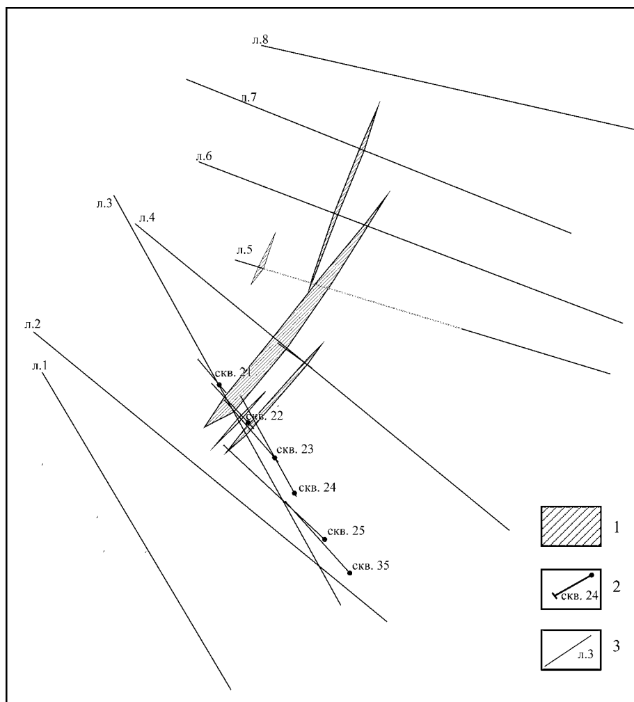
Рис. 2. План по хромитовому месторождению южной части Верх-Нейвинского массива.
