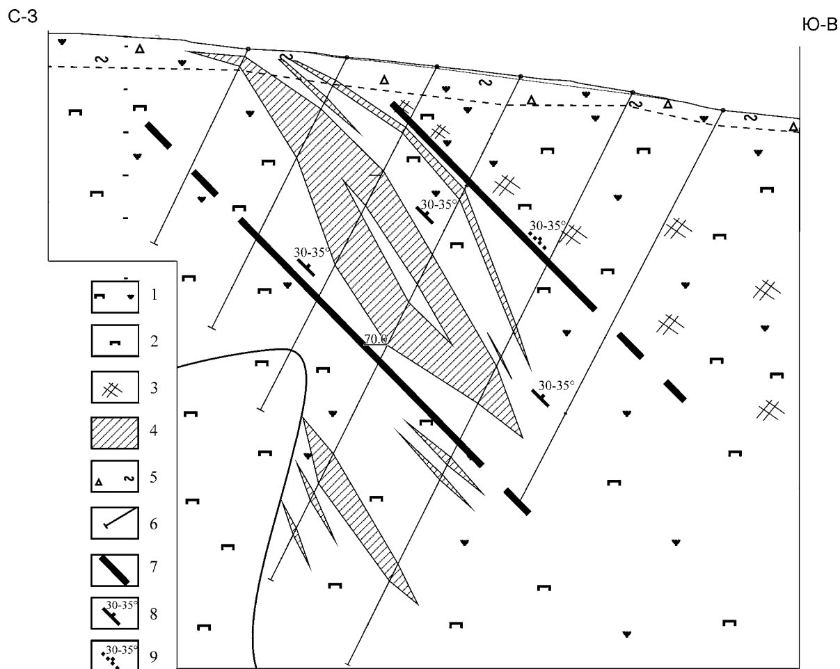
Рис. 1. Разрез (линия 3) по хромитовому месторождению южной части Верх-Нейвинского массива.
